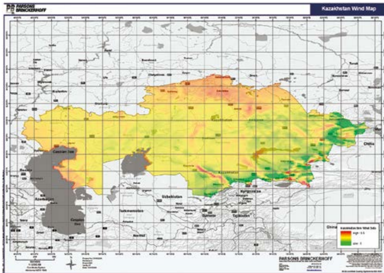
Рисунок 1. Ветровой атлас Казахстана (Источник: Parsons Brinckerhoff) Figure 1. Wind atlas of Kazakhstan (Source: Parsons Brinckerhoff)
